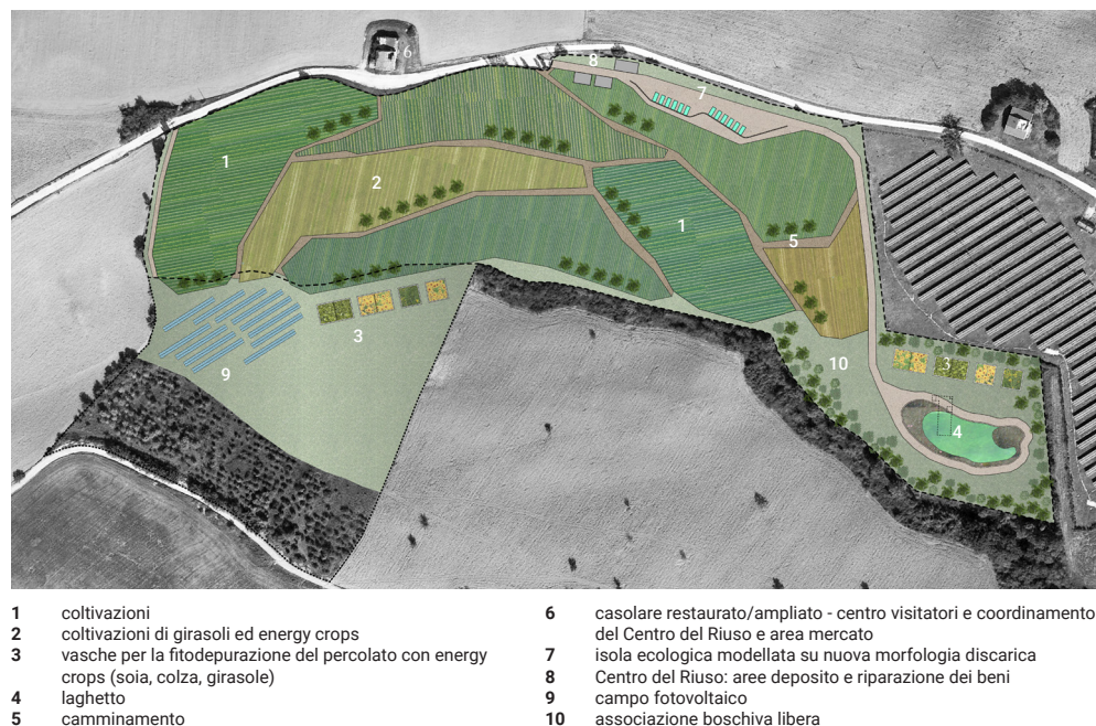
Figura 7.17. Planimetria e disegno generale dell'area. La morfologia della discarica è stata interamente progettata sulla base della planimetria finale. Progetto e grafica: Studio Arcoplan
