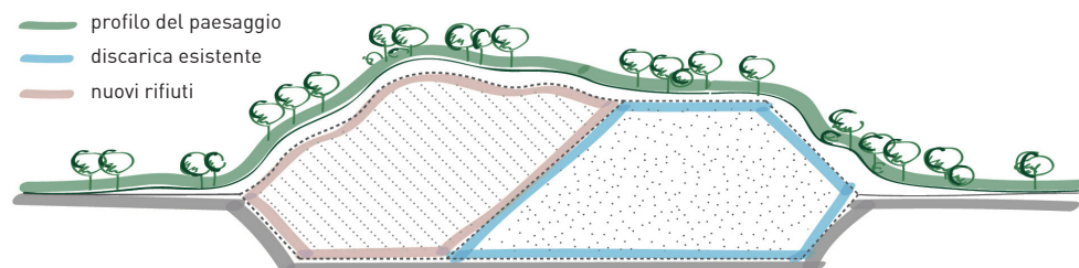
SCENARIO B. Possibilità di intervento nelle discariche ancora in attività, con utilizzo dei rifiuti come materiale plastico per modellare il paesaggio
