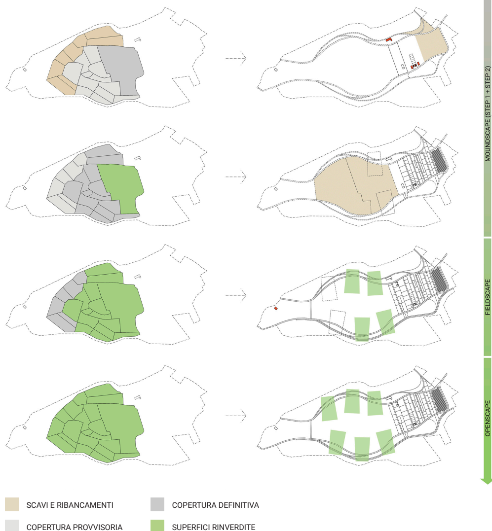
Figura 7.15. Esempio di timeline con programmazione delle attività di abbancamento dei rifiuti in relazione al progressivo utilizzo delle aree. Lo studio cronologico delle diverse soluzioni progettuali mette in relazione la progressione di abbancamento delle terre di scavo e stesura della copertura provvisoria e definitiva, con gli interventi funzionali via via realizzabili. Progetto e Grafica: Studio Arcoplan
