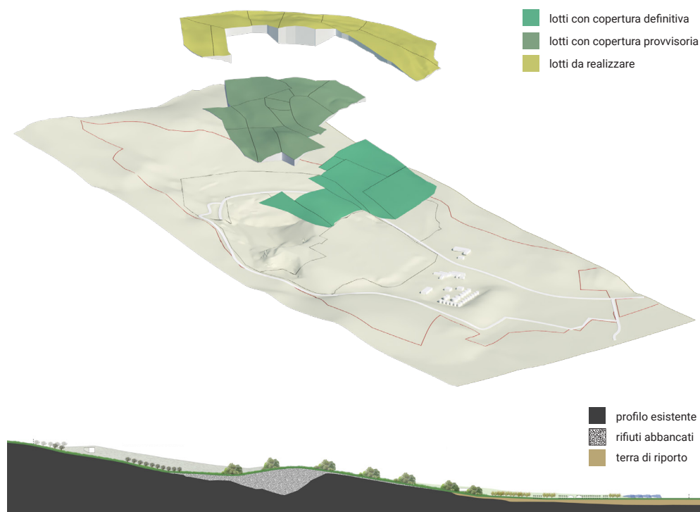
Figura 7.14. Studio dell’inserimento di nuovi volumi in una discarica in ampliamento e sezione trasversale. I nuovi rifiuti abbancati vengono utilizzati come un materiale plastico per sagomare la forma stabilita dal progetto sul paesaggio. Grafica: Studio Arcoplan
