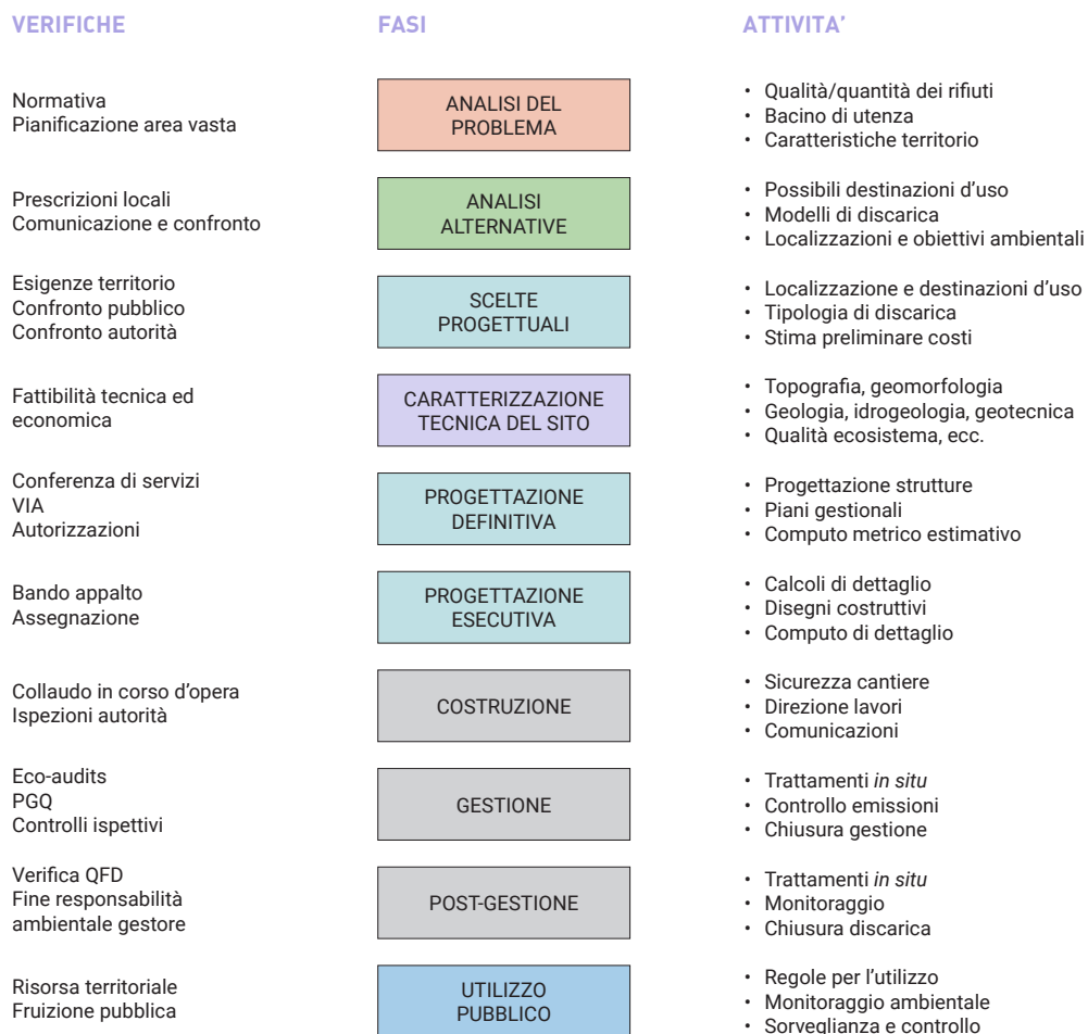
Figura 7.2. Schema delle diverse fasi progettuali di una discarica sostenibile, (modificato da Cossu e Stegmann, 2018).
